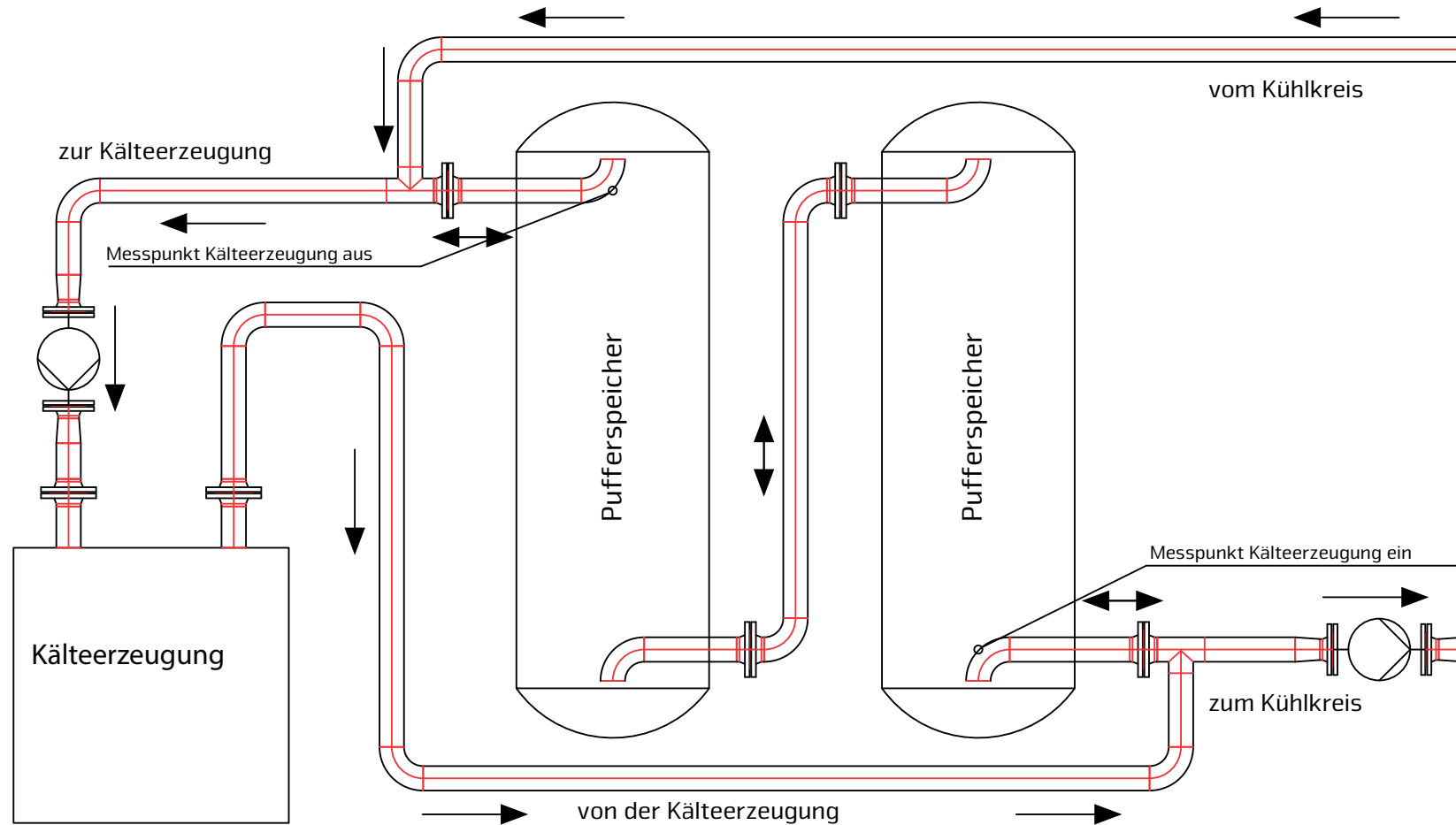
Beispiel der hydraulischen Einbindung einer Pufferbatterie in ein Kaltwassernetz (vereinfachte Darstellung)
