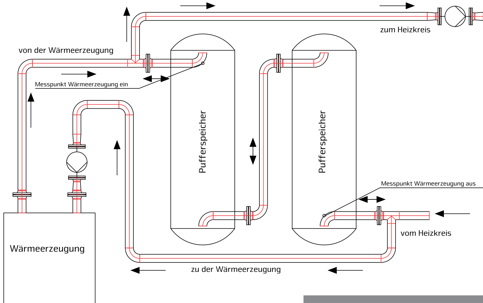
Beispiel der hydraulischen Einbindung einer Pufferbatterie in ein Heizungsnetz (vereinfachte Darstellung)
